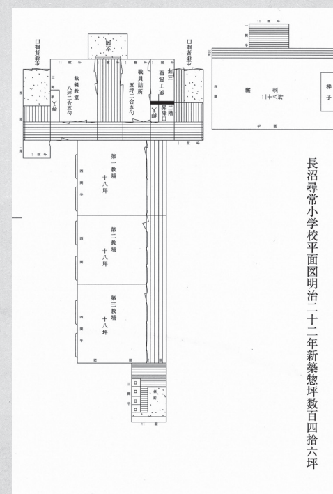
長沼尋常小学校平面図 ([長沼町史 第4巻資料編Ⅲ(上)近代編]より転載)
